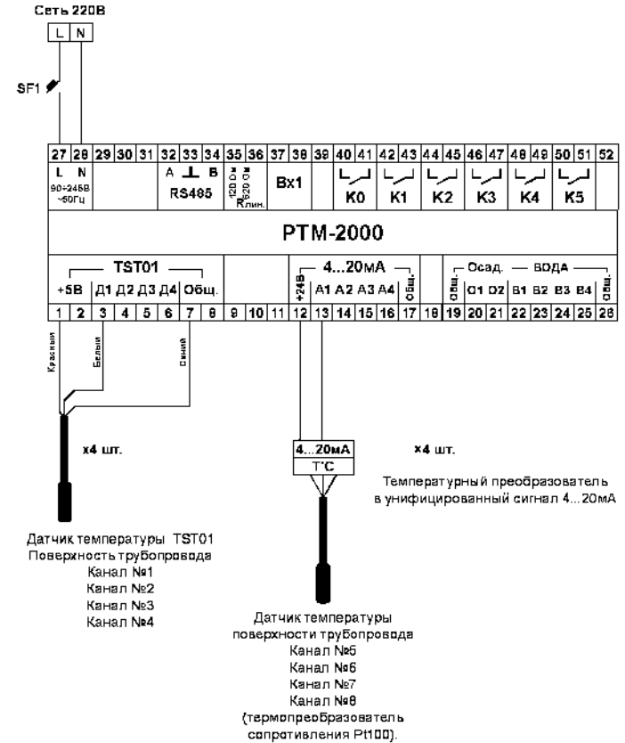
Рис. 23. Типовая схема включения алгоритма «ИЗМЕРИТЕЛЬ».
