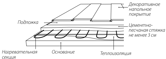
Схема укладки под ламинат, линолеум или ковролин
